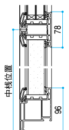
●断熱腰パネル
