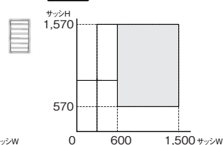
横格子
