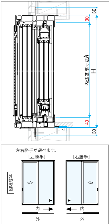
北海道規格 内法基準寸法 h =サッシH-70mm
