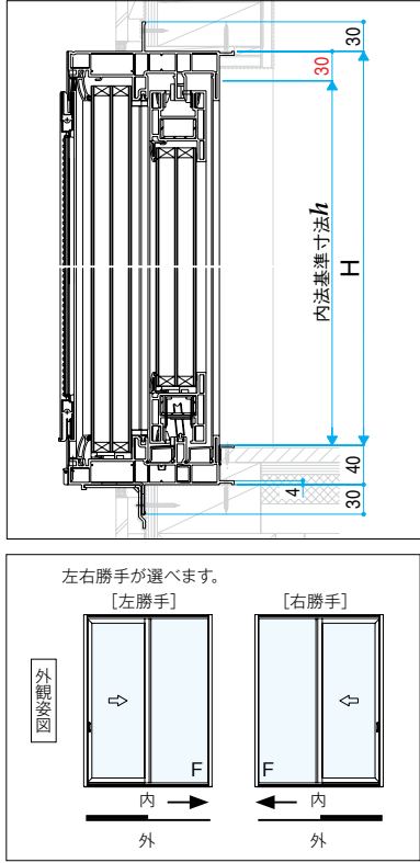
本州規格 内法基準寸法h=サッシH-30mm
