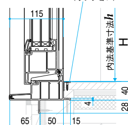
下枠アングル (オプション)
