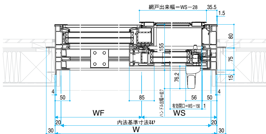
●顔縁納まり
