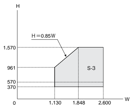
4枚建
