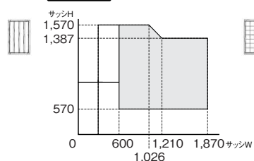
たて格子
