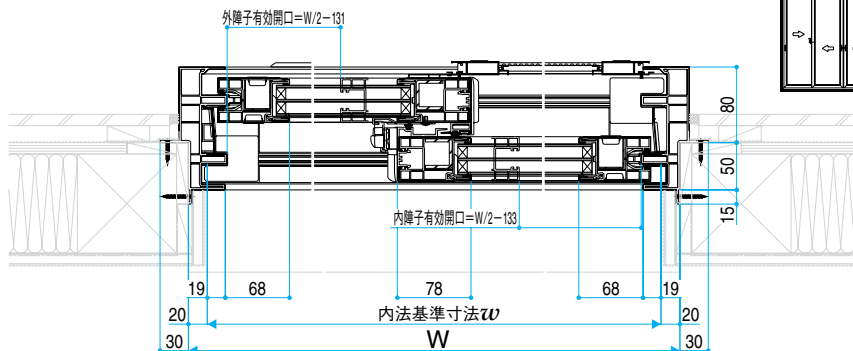
●4枚建
