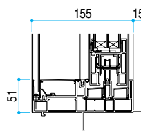
●内障子側(引寄せ前)
