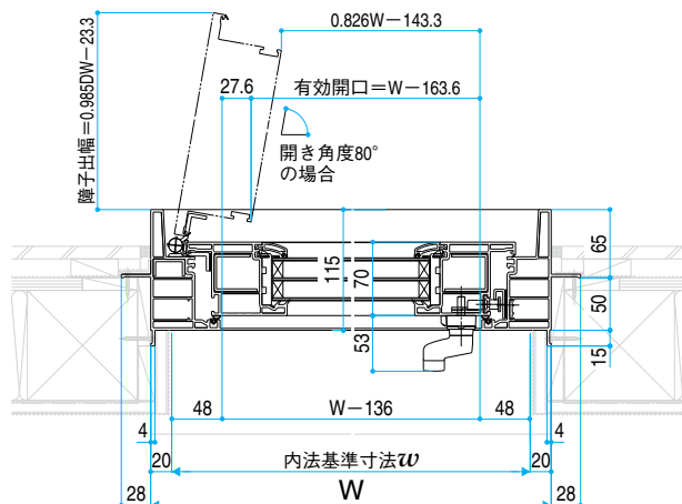
●3連窓
