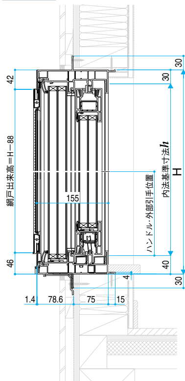
北海道規格/ハンドル・外部引手位置
