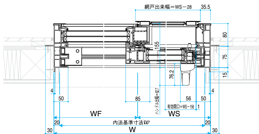
●額縁納まり
