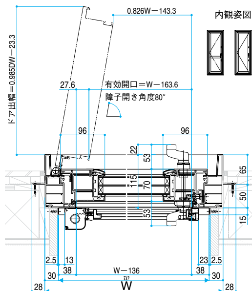
ドア出幅=0.985DW-233.3 0.826W-143.3 有効開口=W-163.6 開き角度80°の場合 DW=W-68 有効開口面積 北海道規格 (W-163.6)×(H-136) 本州規格 (W-163.6)×(H-96) 4 20 28 W-136 内法基準寸法w W 4 20 28 27.6 53 11.5 70 53 39 2 50 15 65 22
