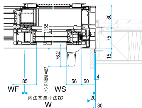
●顔縁納まり
