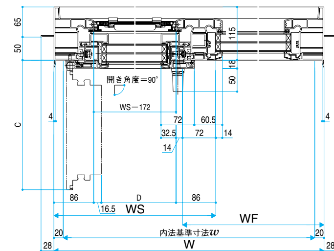
●3連窓
