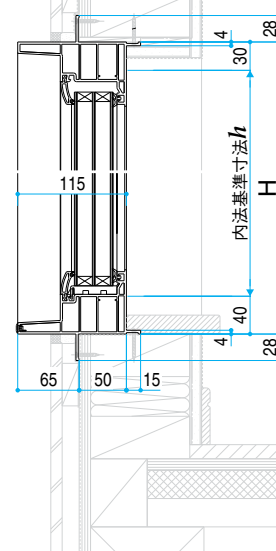
●FIX窓部
