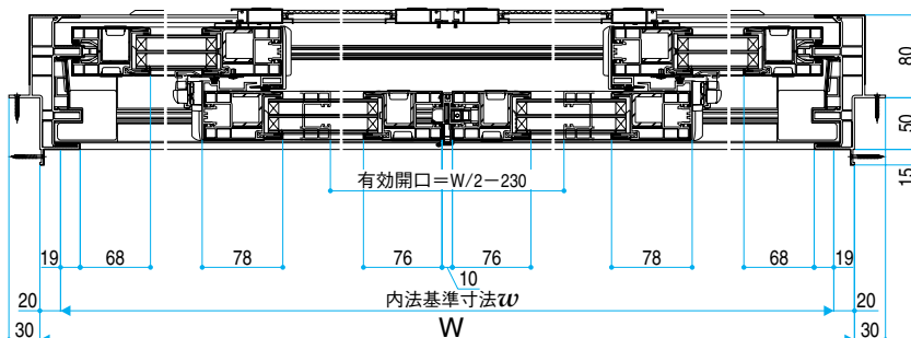
●4枚建
