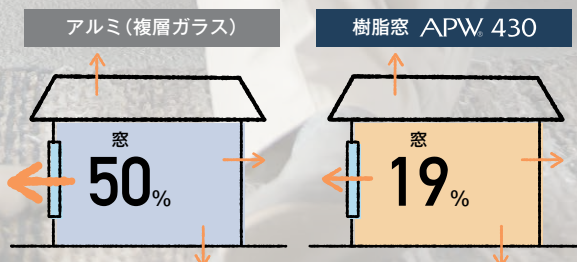
■窓から逃げる熱損失割合比較
